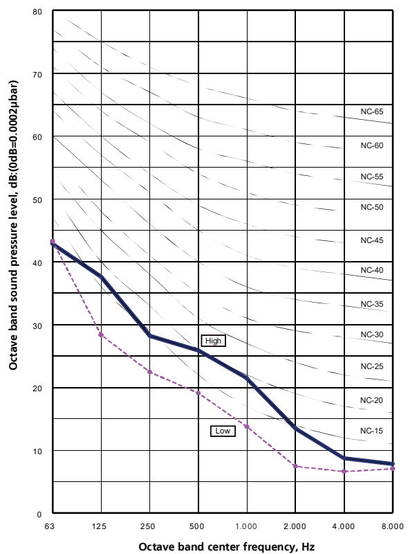
ARXD 14GALH
