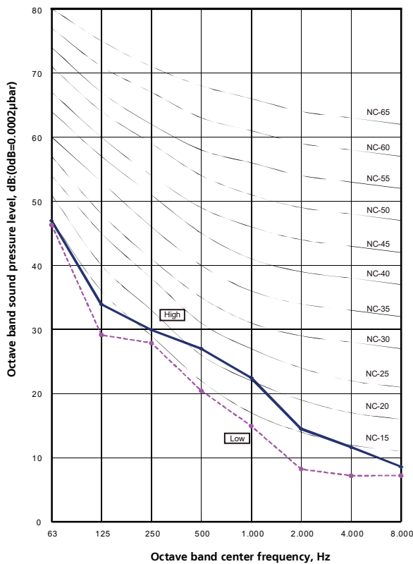
ARXD 12GALH
