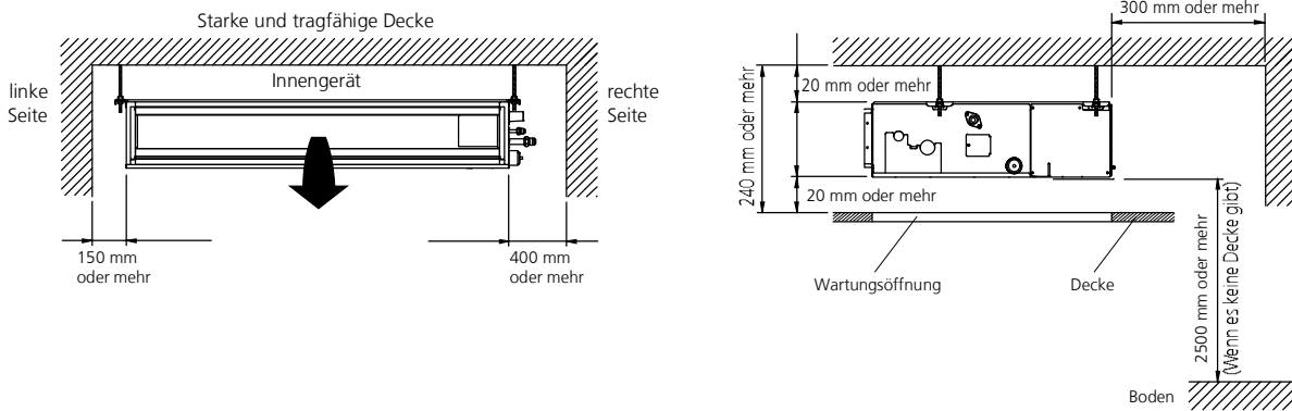
Deckeneinbau
