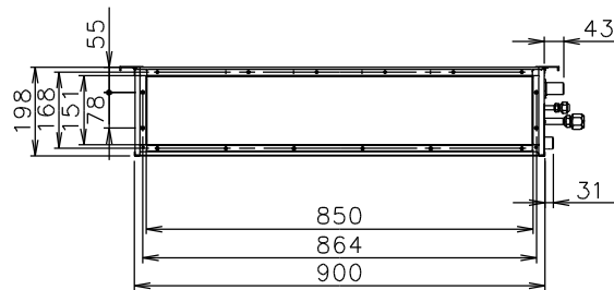
Ausblasseite
